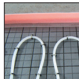
Redumax Kantstrook DUO met vloerverwarming op ThermoTACK.
